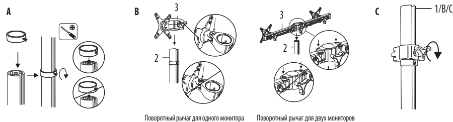
Поворотный рычаг для одного монитора
